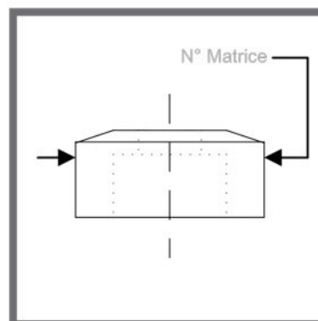
Matrice N°14 Diam: 2 à 8mm
